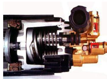
斜盘泵(OTHER)
